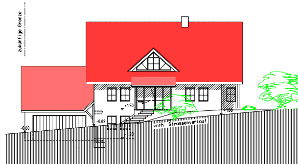
Ansicht West
